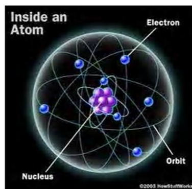
Struktur Atom
